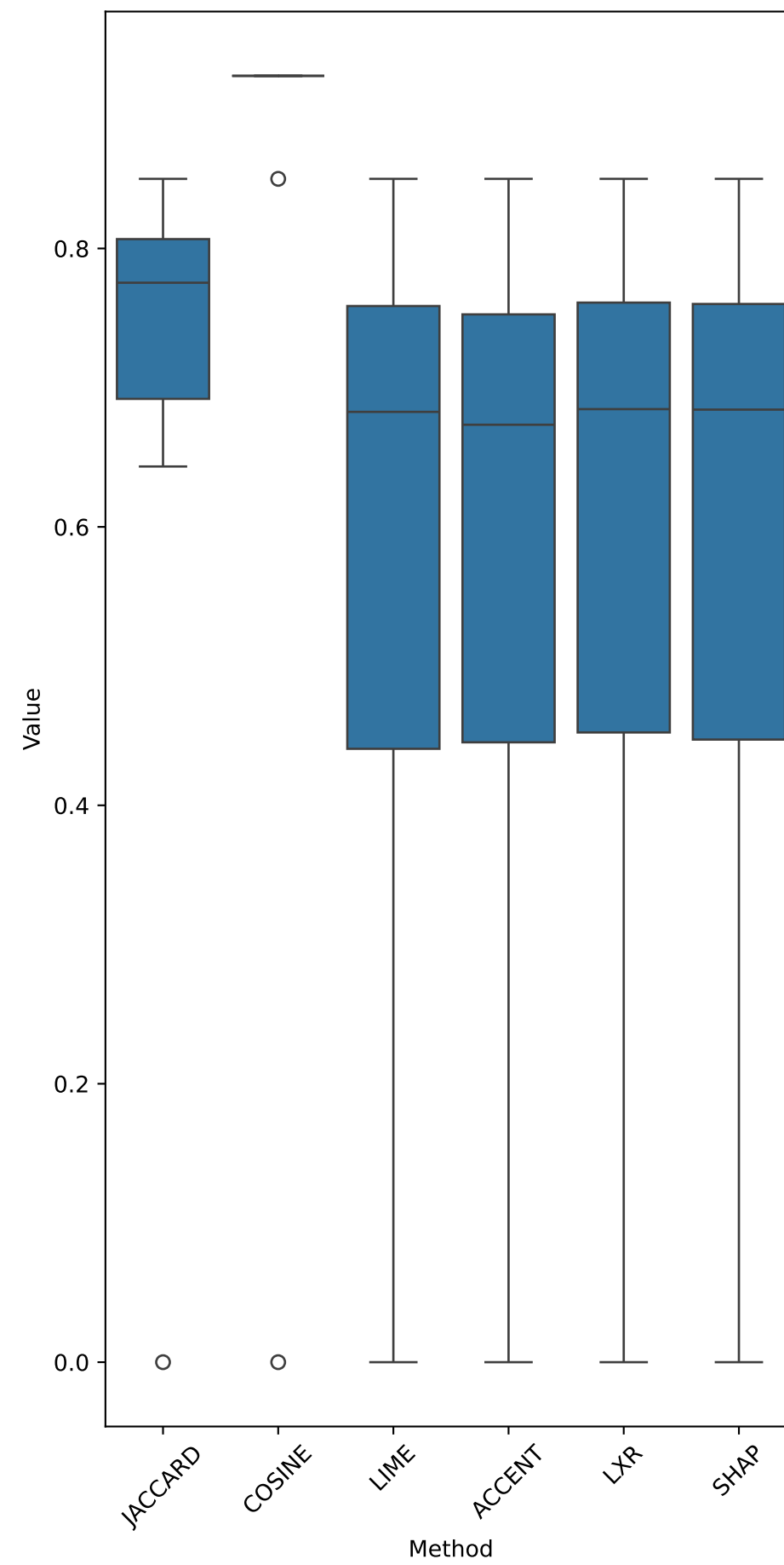
INS Distribution
